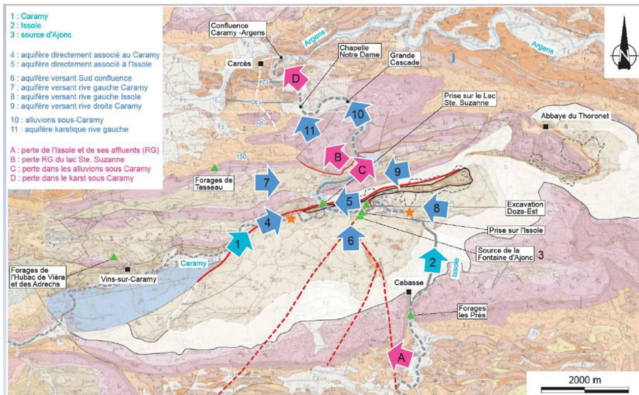
Figure 4 : Zones d'apports et de pertes observées au niveau de la retenue
