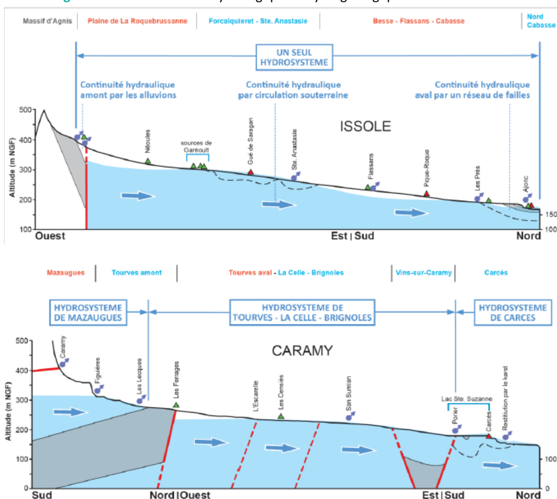
Figure 3 : Fonctionnement hydrologique et hydrogéologique du bassin versant
